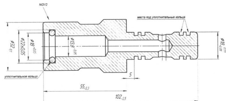
Рисунок 2 – Эскиз изделия
